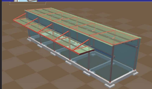
【S造】平屋倉庫（32.5m×8.00m）
