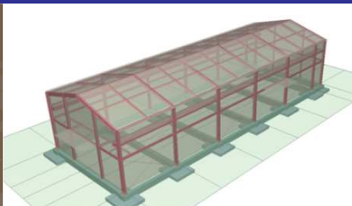
【S造】平屋倉庫（32.0m×10.7m）
